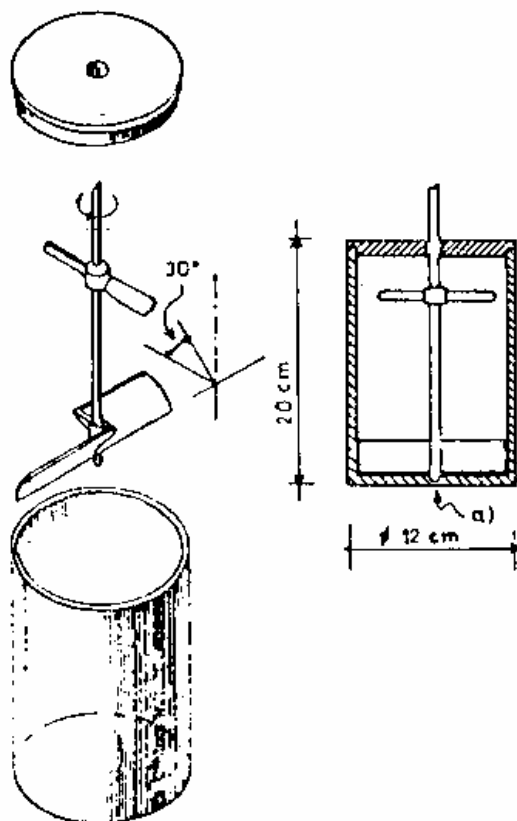
Figura 1 - Estrattore
